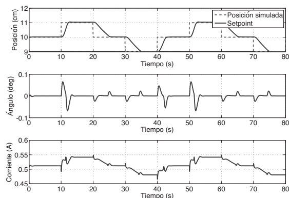
Figura 10: Test de estabilidad 2 seguimiento de referencia escalonadas en el rango [9 – 11]cm con saltos de 1cm.
