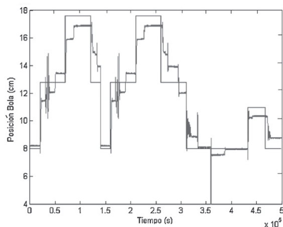
Figura 12: Test de seguimiento escalonado por modos deslizantes.
